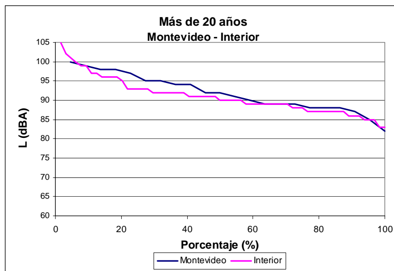
Figura 9. Curvas de excedencia de niveles sonoros de emisión para vehículos de transporte de pasajeros de más de 20 años de antigüedad empadronados en Montevideo y en el interior del país.
