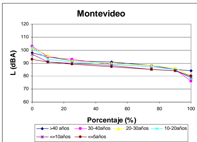
Figura 2. Curvas de excedencia de niveles sonoros de emisión para vehículos de transporte de cargas empadronados en Montevideo, según edad.
