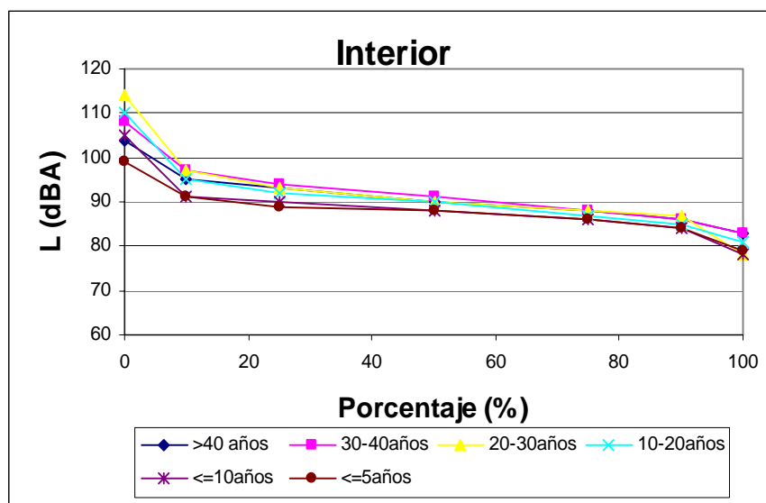
Figura 3. Curvas de excedencia de niveles sonoros de emisión para vehículos de transporte de cargas empadronados en el interior del país, según edad.
